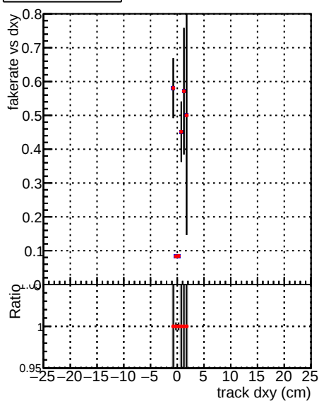
—●— DQM_mkFit_XiMinusPU_retrain2 —●— DQM_mkFit_XiMinusPUold
