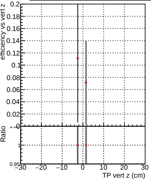
Efficiency vs TP vert z (cm) Legend: DQM_mkFit_XiMinusPU_retrain2 DQM_mkFit_XiMinusPUold
