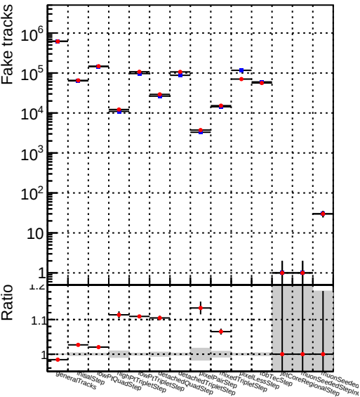
Number —●— DQM_mkFit_XiMinusPUold
