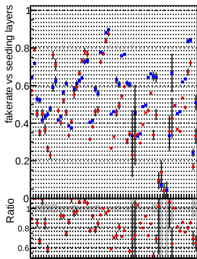
—◆— DQM_mkFit_XiMinusPU_retrain2 —◆— DQM_mkFit_XiMinusPUold
