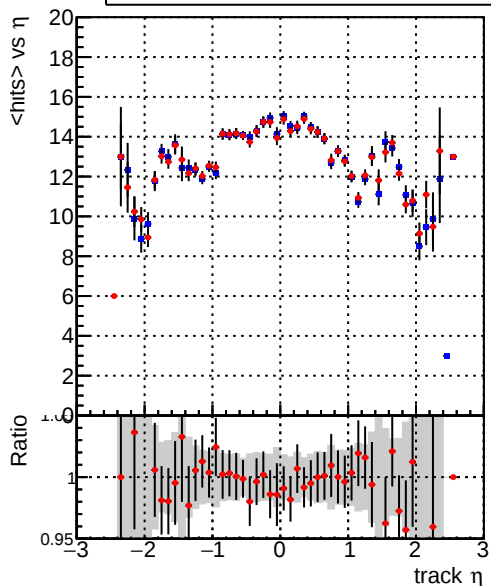
— DQM_mkFit_XiMinusPU_retrain2 — DQM_mkFit_XiMinusPUold mean hits
