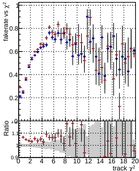
Fake rate vs. —♦— DQM_mkFit_XiMinusPU_retrain2 —●— DQM_mkFit_XiMinusPUold
