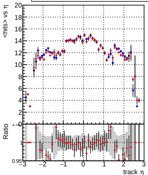
— DQM_mkFit_XiMinusPU_retrain2 — DQM_mkFit_XiMinusPUold mean hits
