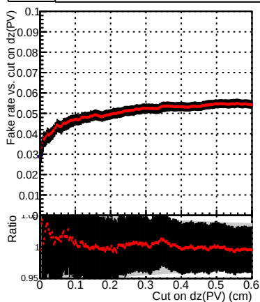
Fake rate —●— DQM_mkFit_XiMinusPUold
