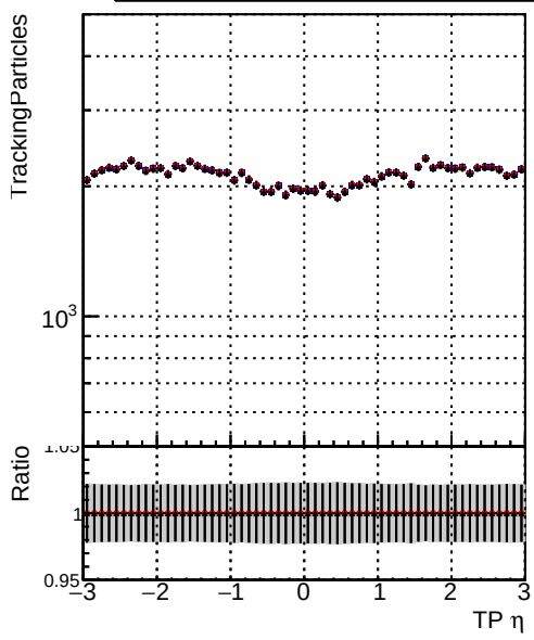
● DQM_mkFit5_XiMinusPUold ● DQM_mkFit5_XiMinusPU_retrain2 ● DQM_mkFit5_XiMinusPU_NEWdefault_specPLess3-2
