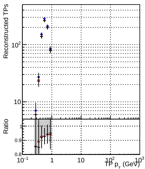
● DQM_mkFit5_XiMinusPUold ● DQM_mkFit_XiMinusPU_retrain2 ● DQM_mkFit_XiMinusPU_NEWdefault_specPLess3-2
