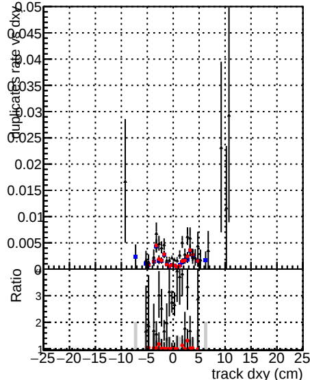
—•— DOM mkFit5 XiMinusPUold —•— DOM mkFit XiMinusPUtrain2 —•— DOM mkFit XiMinusPU NEWdefault specPLESS3-2
