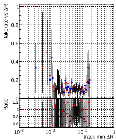
Legend: —•— DQM_mkFit5_XiMinusPUold —•— DQM_mkFit5_XiMinusPU_retrain2 —•— DQM_mkFit5_XiMinusPU_NEWdefault_specPLess3-2
