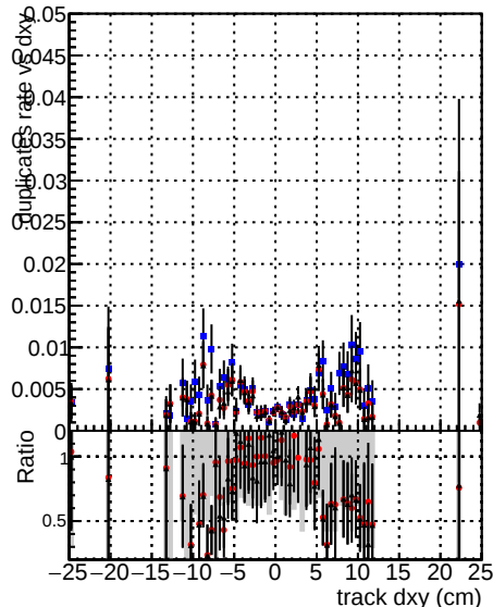
DOM mkFit5 XiMinusPUold DOM mkFit5 XiMinusPU XiMinusPU DOM mkFit5 XiMinusPU NEWdefault specPLESS3-2
