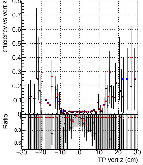
Efficiency vs. TP vert z —●— DQM_mkFit5_XiMinusPUold —●— DQM_mkFit_XiMinusPU_retrain2 —●— DQM_mkFit_XiMinusPU_NEWdefault_specPless3-2
