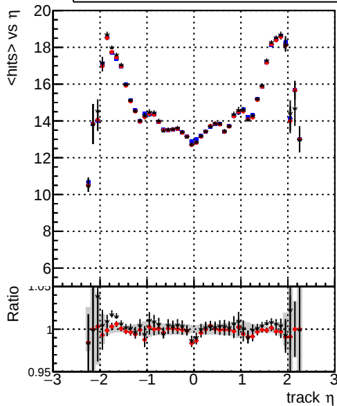
mean hit — DQM_mkFit5_XiMinusPUold — DQM_mkFit5_XiMinusPU_retrain2 — DQM_mkFit5_XiMinusPU_NEWdefault_specPLess3-2
