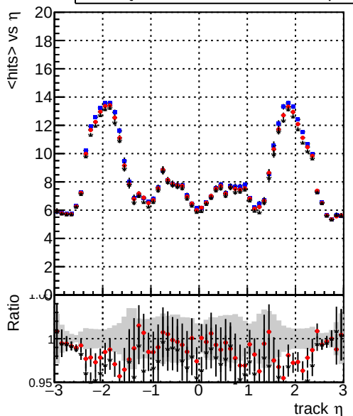
— DQM_mkFit5_XiMinusPUold — DQM_mkFit5_XiMinusPU_retrain2 — DQM_mkFit5_XiMinusPU_NEWdefault_specPLess3-2 mean hit
