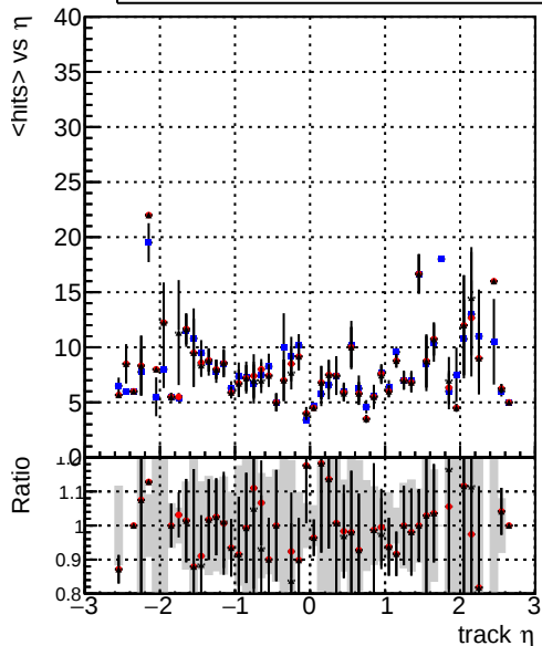
mean hit — DQM_mkFit5_XiMinusPUold — DQM_mkFit_XiMinusPU_retrain2 — DQM_mkFit_XiMinusPU_NEWdefault_specPless3-2
