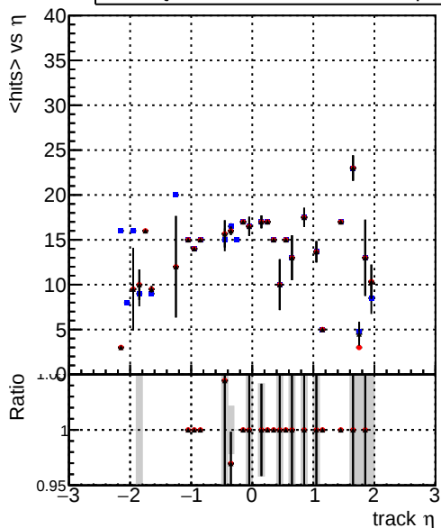
mean hit — DQM_mkFit5_XiMinusPUold — DQM_mkFit5_XiMinusPU_retrain2 — DQM_mkFit5_XiMinusPU_NEWdefault_specPLess3-2
