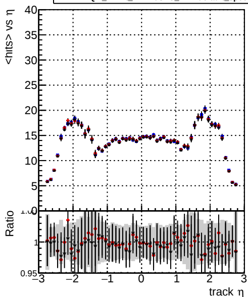
mean hit — DQM_mkFit5_XiMinusPUold — DQM_mkFit_XiMinusPU_retrain2 — DQM_mkFit_XiMinusPU_NEWdefault_specPLess3-2
