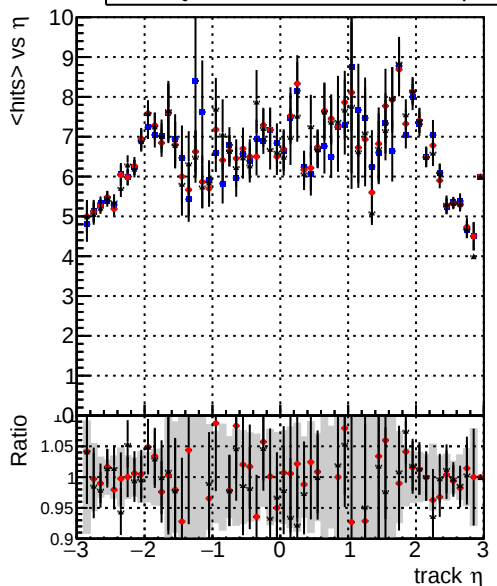
mean hit — DQM_mkFit5_XiMinusPUold — DQM_mkFit5_XiMinusPU_retrain2 — DQM_mkFit5_XiMinusPU_NEWdefault_specPLess3-2
