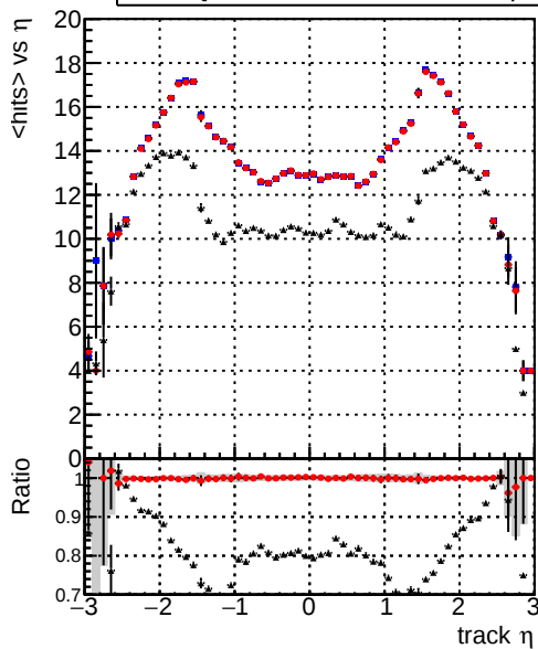
— DQM_mkFit5_XiMinusPUold — DQM_mkFit_XiMinusPU_retrain2 — DQM_mkFit_XiMinusPU_NEWdefault_specPLess3-2 mean hit
