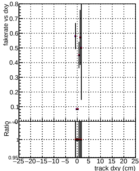
DOM mkFit5 XiMinusPUold DOM mkFit5 XiMinusPUold DOM mkFit5 XiMinusPUold
