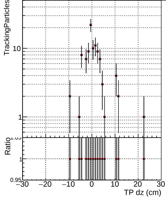
N of simulated track DQM_mkFit5_XiMinusPUold DQM_mkFit_XiMinusPU_retrain2 DQM_mkFit_XiMinusPU_NEWdefault_specPLess3-2
