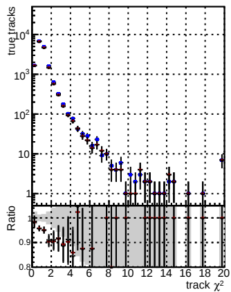
N of reco track vs. \chi^2 DQM mFit XiMinusPUbold DQM mFit XiMinusPU retrain2 DQM mFit XiMinusPU NEWdefault specPLess3-2
