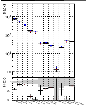
N of reco track vs. \chi^2 DQM mFit XiMinusPUbold DQM mFit XiMinusPU retrain2 DQM mFit XiMinusPU NEWdefault specPLess3-2
