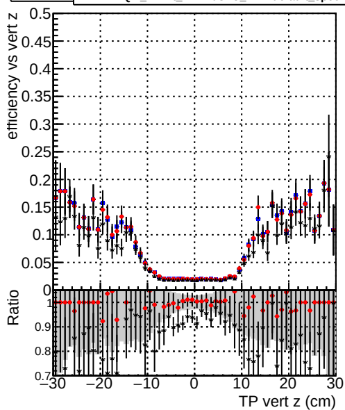
Efficiency vs. sim PV z — DQM_mkFit5_XiMinusPUold — DQM_mkFit_XiMinusPU_retrain2 — DQM_mkFit_XiMinusPU_NEWdefault_specPless3-2
