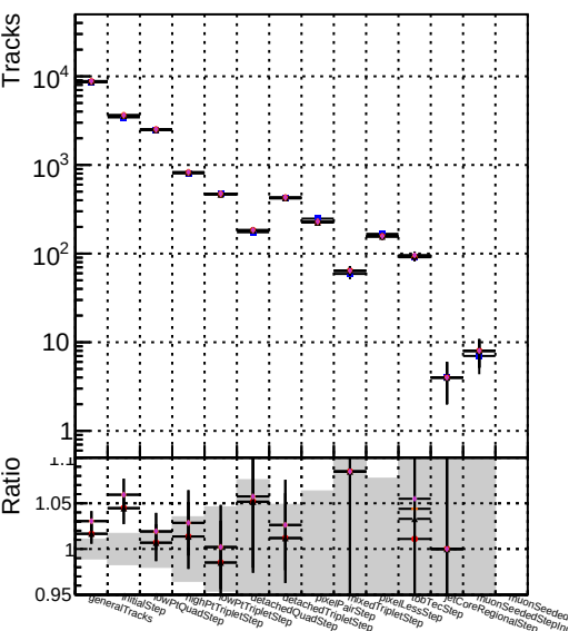
DOM mkFit XiMinus PU retrain-lowpt specPLess1-lowpt DOM mkFit XiMinus PU NEWdefault specPLess2-lowpt DOM mkFit XiMinus PU NEWdefault specPLess3-lowpt DOM mkFit XiMinus PU NEWdefault specPLess4-lowpt
