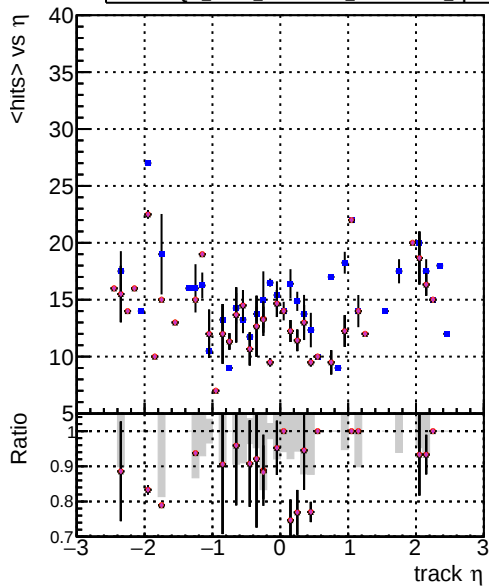
Legend: — DQM mkFit XiMinusPU tetaInLowpt specPless1-lowpt — DQM mkFit XiMinusPU NEWdefault specPless2-lowpt — DQM mkFit XiMinusPU NEWdefault specPless3-lowpt — DQM mkFit XiMinusPU NEWdefault specPless4-lowpt
