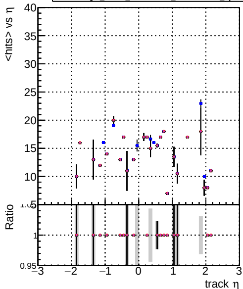
Legend: DQM mkFit XiMinusPU ttrain-lowpt, DQM mkFit XiMinusPU NEWdefault specLess1-lowpt, DQM mkFit XiMinusPU NEWdefault specLess2-lowpt, DQM mkFit XiMinusPU NEWdefault specLess3-lowpt, DQM mkFit XiMinusPU NEWdefault specLess4-lowpt mean hits
