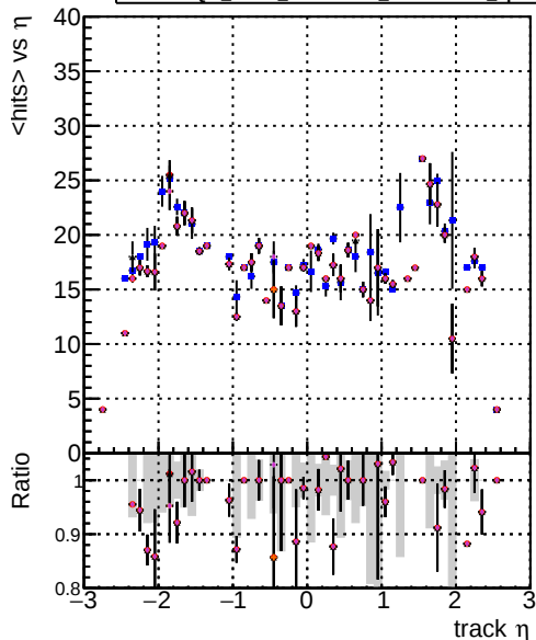
mean hit DQM mkFit XiMinusPU NEWdefault specPLess1-lowpt DQM mkFit XiMinusPU NEWdefault specPLess2-lowpt DQM mkFit XiMinusPU NEWdefault specPLess3-lowpt DQM mkFit XiMinusPU NEWdefault specPLess4-lowpt
