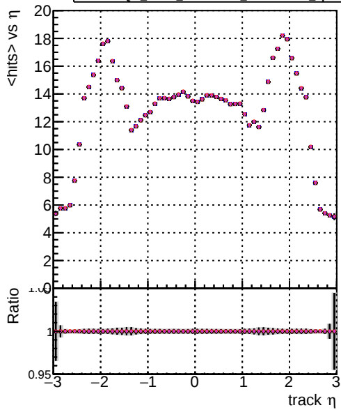
mean hit DQM mkFit XiMinusPU tetrailowpt specPless1-lowpt DQM mkFit XiMinusPU NEWdefault specPless2-lowpt DQM mkFit XiMinusPU NEWdefault specPless3-lowpt DQM mkFit XiMinusPU NEWdefault specPless4-lowpt
