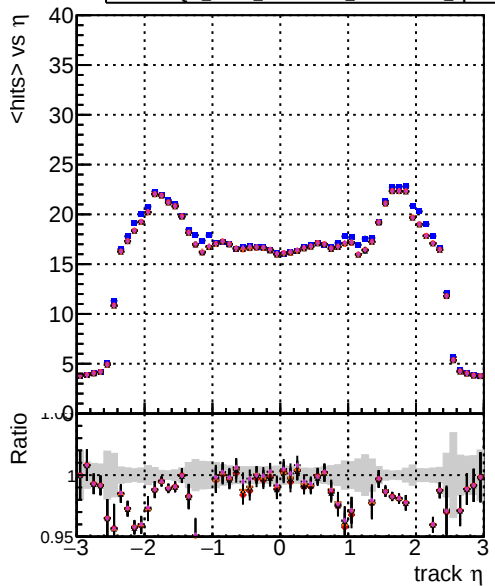
mean hit DQM mkFit XiMinusPU NEWdefault specPless1-lowpt DQM mkFit XiMinusPU NEWdefault specPless2-lowpt DQM mkFit XiMinusPU NEWdefault specPless3-lowpt DQM mkFit XiMinusPU NEWdefault specPless4-lowpt
