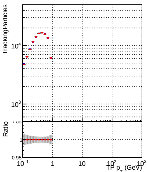
—•— DQM_mkFit_XiMinusPU_retrain2-lowpt —•— DQM_mkFit_XiMinusPUold-lowpt
