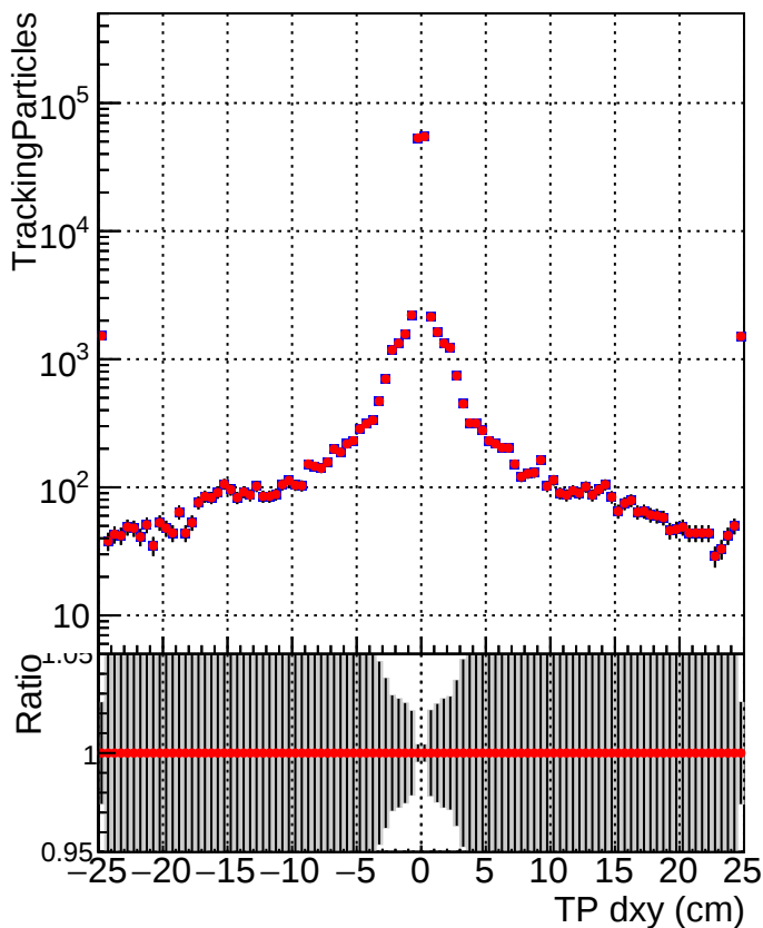
■ DQM_mkFit_XiMinusPU_retrain2-lowpt ● DQM_mkFit_XiMinusPUold-lowpt
