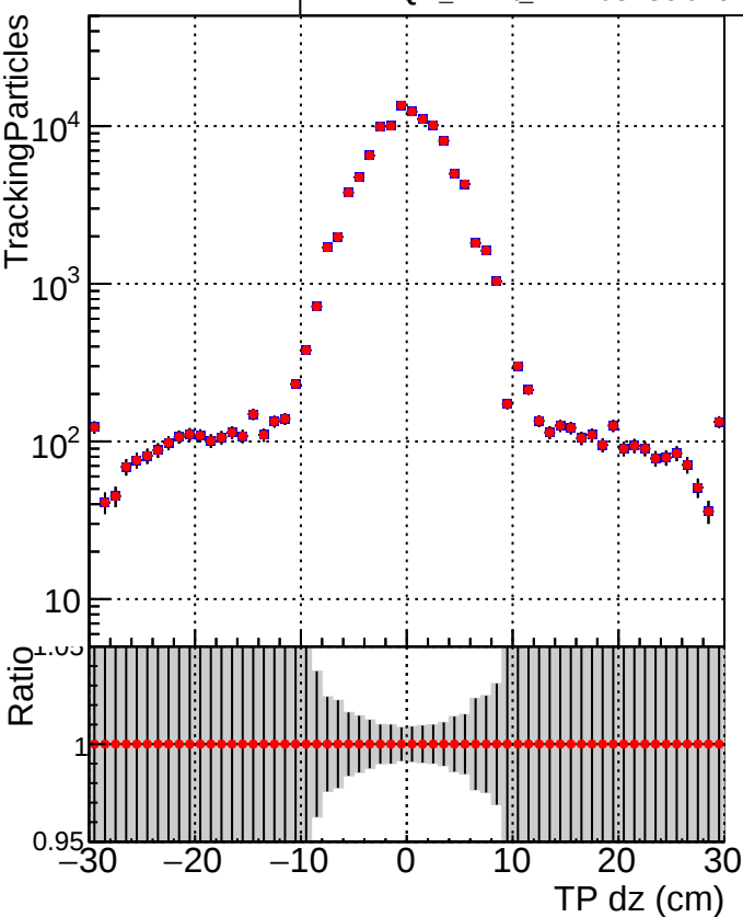
■ DQM_mkFit_XiMinusPU_retrain2-lowpt ● DQM_mkFit_XiMinusPUold-lowpt
