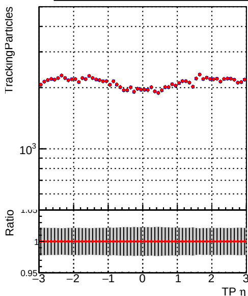
—•— DQM_mkFit_XiMinusPU_retrain2-lowpt —•— DQM_mkFit_XiMinusPUold-lowpt
