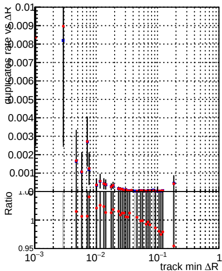
—●— DQM_mkFit_XiMinusPU_retrain2-lowpt —●— DQM_mkFit_XiMinusPUold-lowpt
