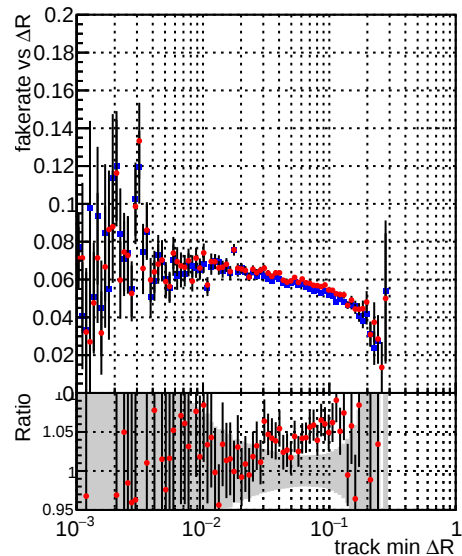
—●— DQM_mkFit_XiMinusPU_retrain2-lowpt —●— DQM_mkFit_XiMinusPUold-lowpt
