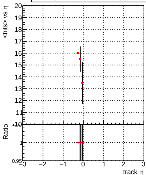
—•— DQM_mkFit_XiMinusPU_retrain2-lowpt —•— DQM_mkFit_XiMinusPUold-lowpt
