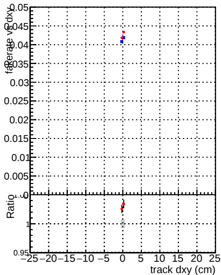
—●— DQM_mkFit_XiMinusPU_retrain2-lowpt —●— DQM_mkFit_XiMinusPUold-lowpt
