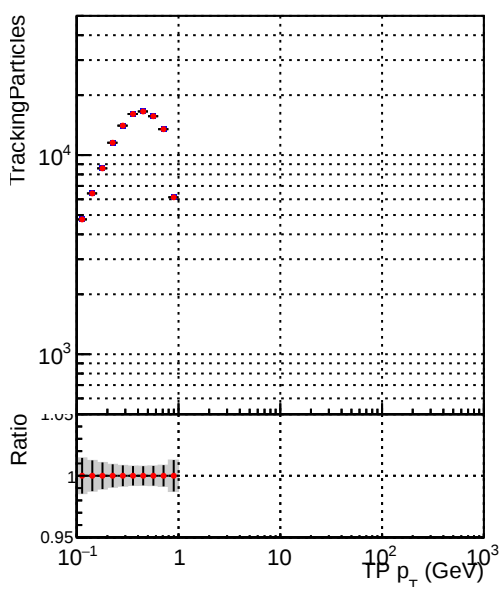
—●— DQM_mkFit_XiMinusPU_retrain2-lowpt —●— DQM_mkFit_XiMinusPUold-lowpt
