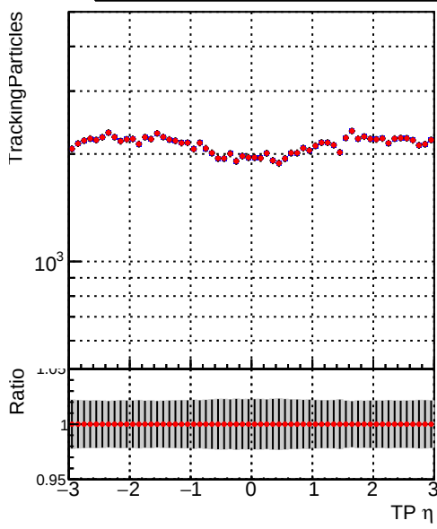
—●— DQM_mkFit_XiMinusPU_retrain2-lowpt —●— DQM_mkFit_XiMinusPUold-lowpt
