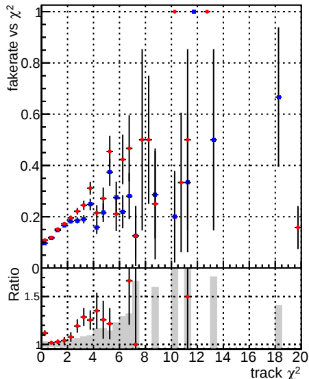
Fake rate vs. —•— DQM_mkFit_XiMinusPU_retrain2-lowpt —•— DQM_mkFit_XiMinusPUold-lowpt
