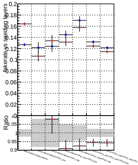
Fake rate vs. —•— DQM_mkFit_XiMinusPU_retrain2-lowpt —•— DQM_mkFit_XiMinusPUold-lowpt
