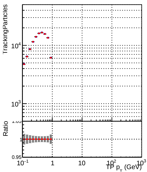
■ DQM_mkFit_XiMinusPU_retrain2-lowpt ■ DQM_mkFit_XiMinusPUold-lowpt
