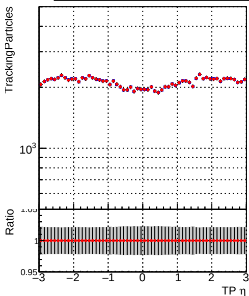
■ DQM_mkFit_XiMinusPU_retrain2-lowpt ■ DQM_mkFit_XiMinusPUold-lowpt
