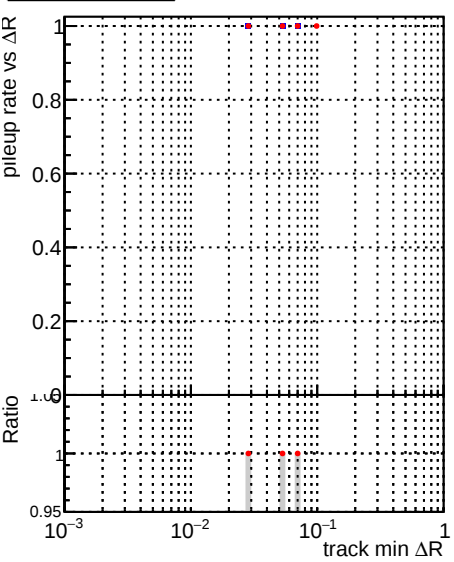
Legend: DQM_mkFit_XiMinusPU_retrain2-lowpt DQM_mkFit_XiMinusPUold-lowpt
