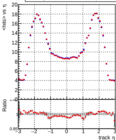
— DQM_mkFit_XiMinusPU_retrain2-lowpt — DQM_mkFit_XiMinusPUold-lowpt
