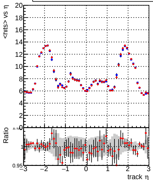
mean hit — DQM_mkFit_XiMinusPU_retrain2-lowpt — DQM_mkFit_XiMinusPUold-lowpt
