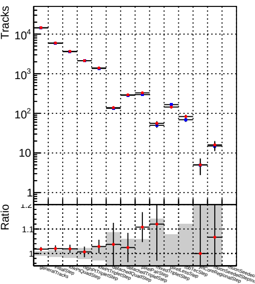
■ DQM_mkFit_XiMinusPU_retrain2-lowpt
