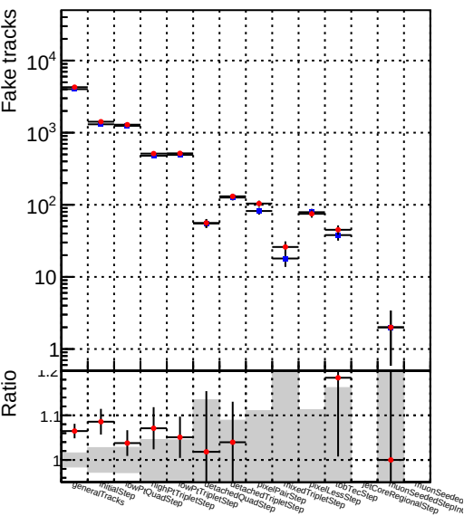
Number —●— DQM_mkFit_XiMinusPUold-lowpt
