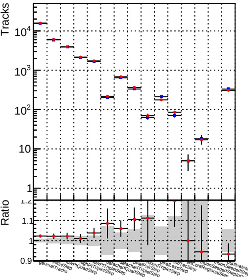
■ DQM_mkFit_XiMinusPU_retrain2-lowpt
