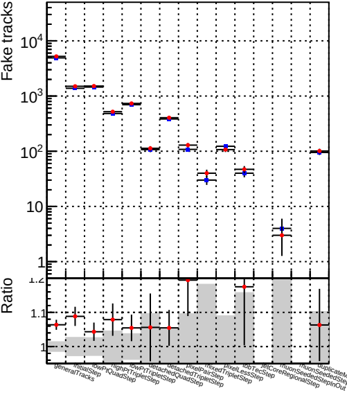
Number —●— DQM_mkFit XiMinusPUold-lowpt
