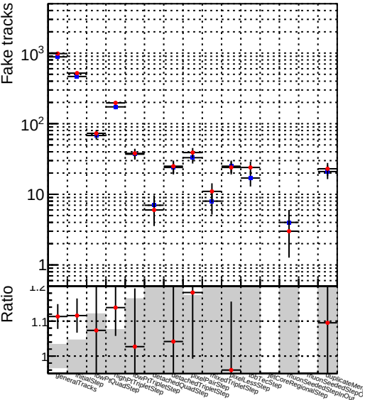
Number —●— DQM_mkFit_XiMinusPUold-lowpt
