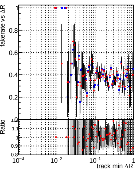
DQM_mkFit_XiMinusPU_retrain2-lowpt DQM_mkFit_XiMinusPUold-lowpt
