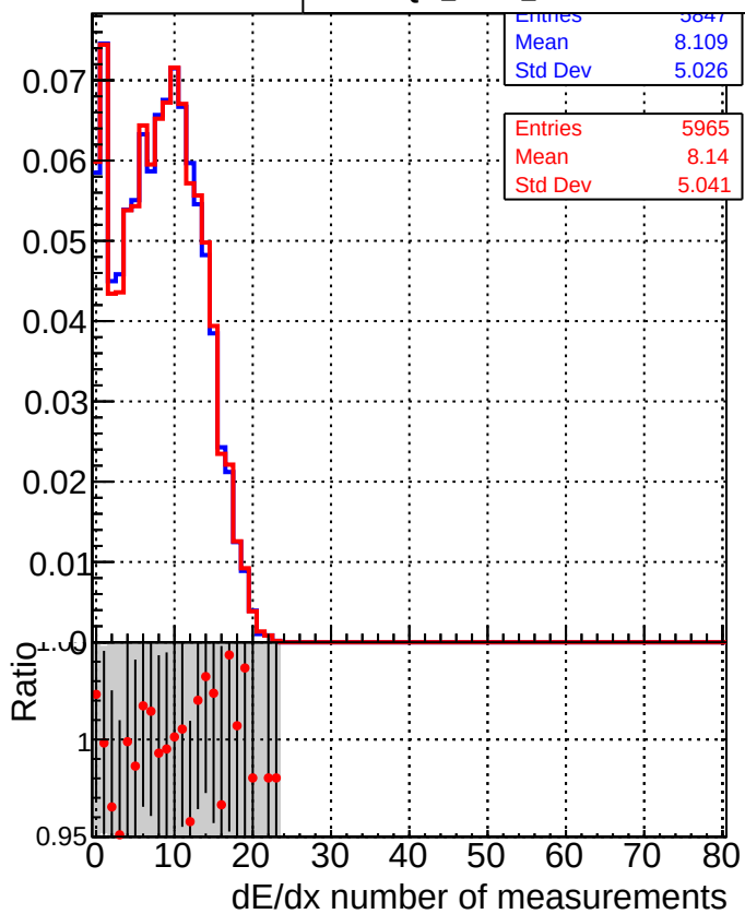
DQM_mkFit_XiMinusPU_retrain2-lowpt DQM_mkFit_XiMinusPUold-lowpt
