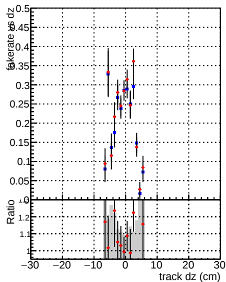
—●— DQM_mkFit_XiMinusPU_retrain2-lowpnt —●— DQM_mkFit_XiMinusPUold-lowpnt
