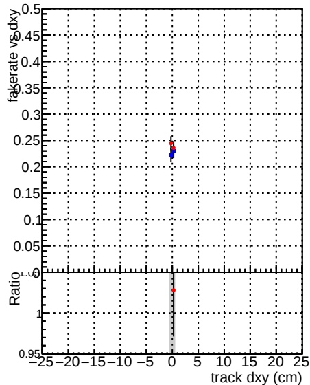
—●— DQM_mkFit_XiMinusPU_retrain2-lowpnt —●— DQM_mkFit_XiMinusPUold-lowpnt
