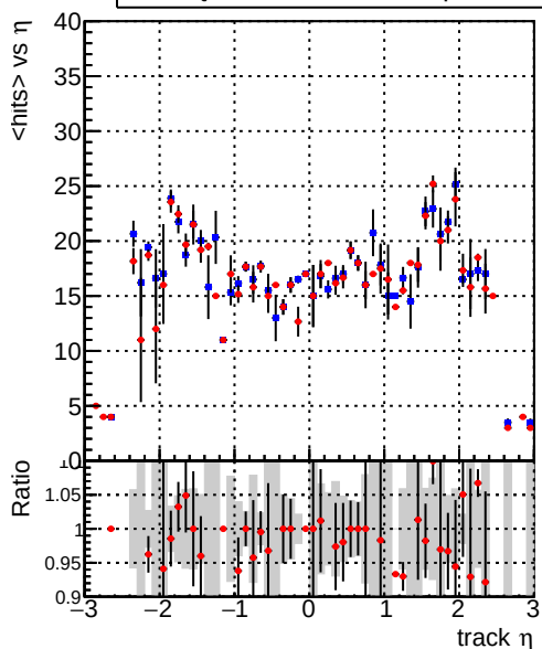
mean hits — DQM_mkFit_XiMinusPU_retrain2-lowpt — DQM_mkFit_XiMinusPUold-lowpt
